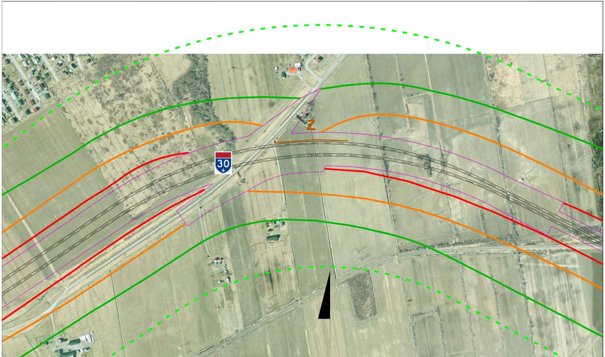
Nouvelle autoroute 30 CJV Figure 8 : Écran antibruit Z
