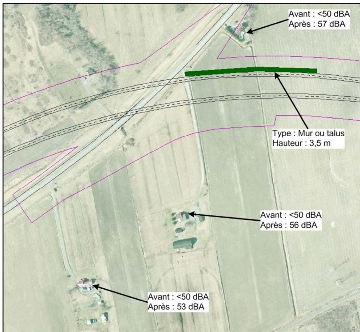
Écran antibruit Z
