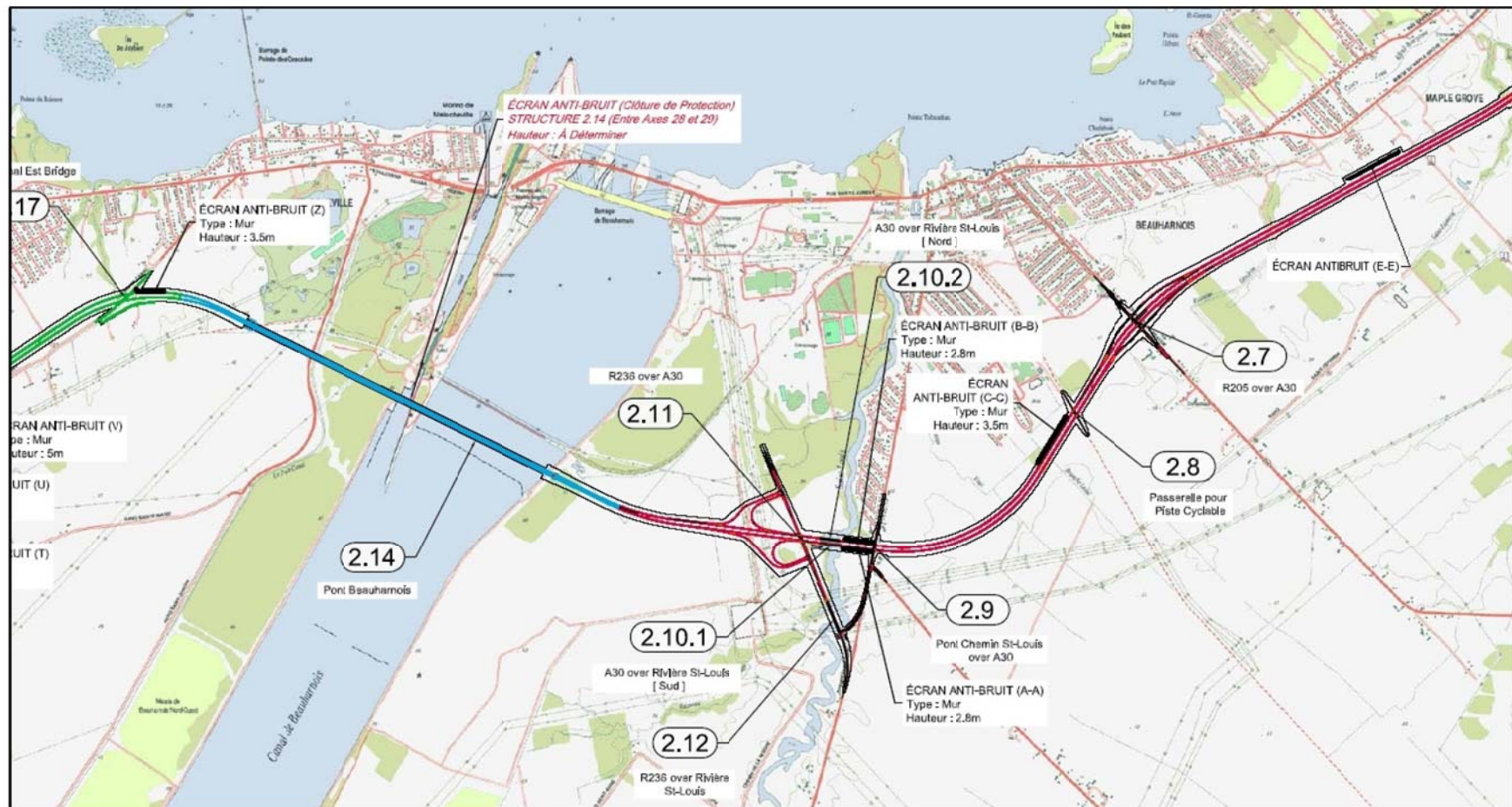
Figure 7 : Emplacement des écrans antibruit
